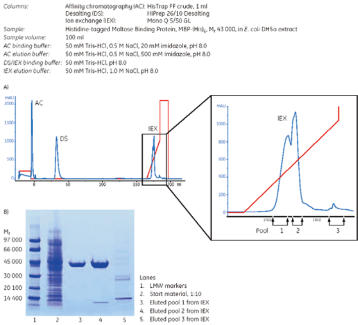
图50：（A）AC—DS—IEX的纯化结果。IEX的峰图的放大版和收集的组分显示在右侧。产率：在收集组分1和2中总共有9.4mg蛋白。（B）从IEX上洗脱的收集组分的SDS-PAGE电泳结果。胶用考马斯亮蓝染色。
