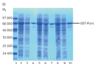
图64: GST-Pur \alpha 蛋白的纯化和规模化放大 (A) GSTrap FF 1ml, (B) GSTrap FF 5ml, (C) GSTPrep16/10, (D) 用Excel Gel (12.5%均一浓度) 胶的SDS-PAGE分析。采用Multiphor II 电泳装置, 考马斯亮蓝染色。由于GST的相对慢结合、低转化率和高上样量, 有些上样的蛋白发现在穿透中。
