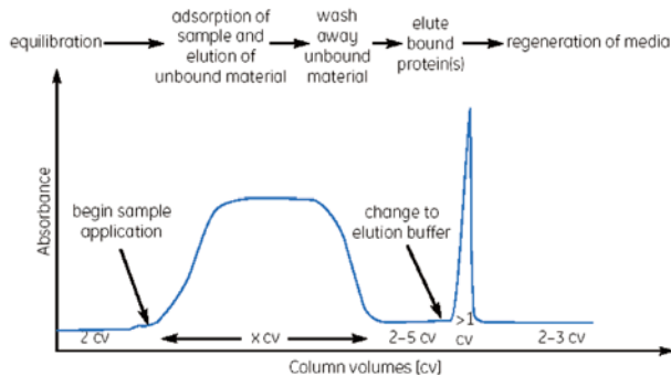
图98：典型的亲和纯化过程。
