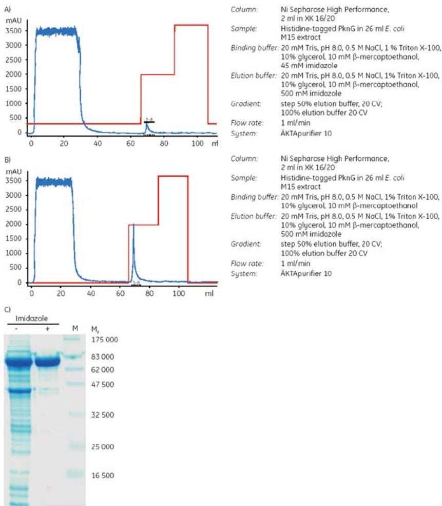
图45：在样品和结合缓冲液中有（A）和没有（B）45mM咪唑的情况下对His6-PknG的纯化。对于每次层析，从2升的大肠杆菌培养物中获得的26ml裂解物用0.45 \mu m滤膜过滤后上样到2ml Ni Sepharose High Performnce（XK16/20柱），层析过程使用ÄKTApurifier。蛋白质激酶用50%和100%的洗脱缓冲液进行两步梯度洗脱。（C）12% SDS-PAGE 检测His6-PknG洗脱组分。（+）表示加入45mM咪唑的结果（-）表示没有加入咪唑的结果。
