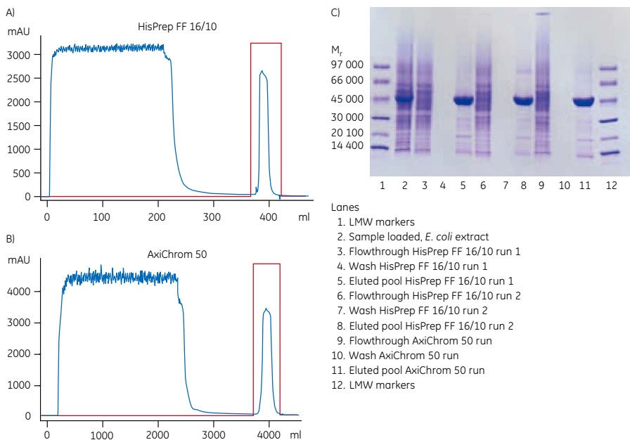
图22：从A（20ml HisPrep FF16/10柱）到B（210ml AxiChromTM50柱）的规模化放大。ÄKTA explorer 100用于进行在HisPrep FF16/10上的纯化，ÄKTA Pilot用于进行在AxiChrom50上的纯化。所有的系统都用UNICORN软件控制。注意，只有一次在HisPrep FF16/10上的运行展示出来。C，SDS-PAGE检测两种纯化的各种组分。
