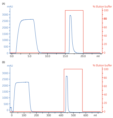
图6.7 MBP2*- \beta -半乳糖苷酶纯化的规模放大，（A）MBPTrap HP 1 ml毫升，（B）Dextrin Sepharose High Performance 的XK 26/20，29毫升。MBPTrap HP 5 ml毫升柱子的色谱图没有显示。
